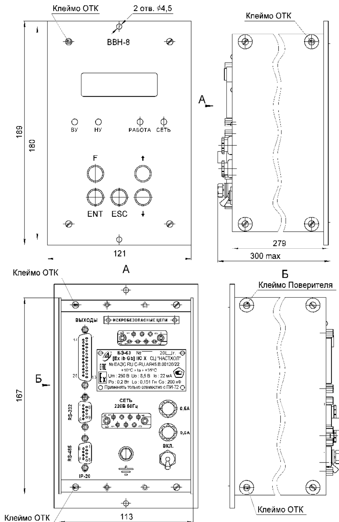
Рисунок А.3 – Внешний вид и габаритные размеры блока БЗ-63 вискозиметра
